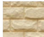
Бежевый
